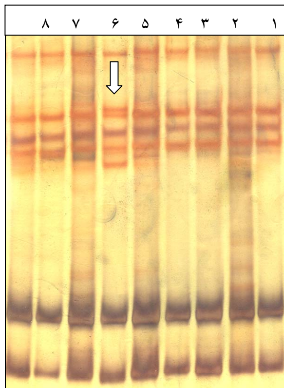
شکل ۱. نمونه ای از ژل SSCP در مورد اگزون ۴ ژن CFTR. ستون ۱ نمونه فرد طبیعی، ستون های ۲-۹ نمونه بیمار. ستون ۴ نشان دهنده جهش 406-6T > C به حالت هتروزیگوت می باشد.
