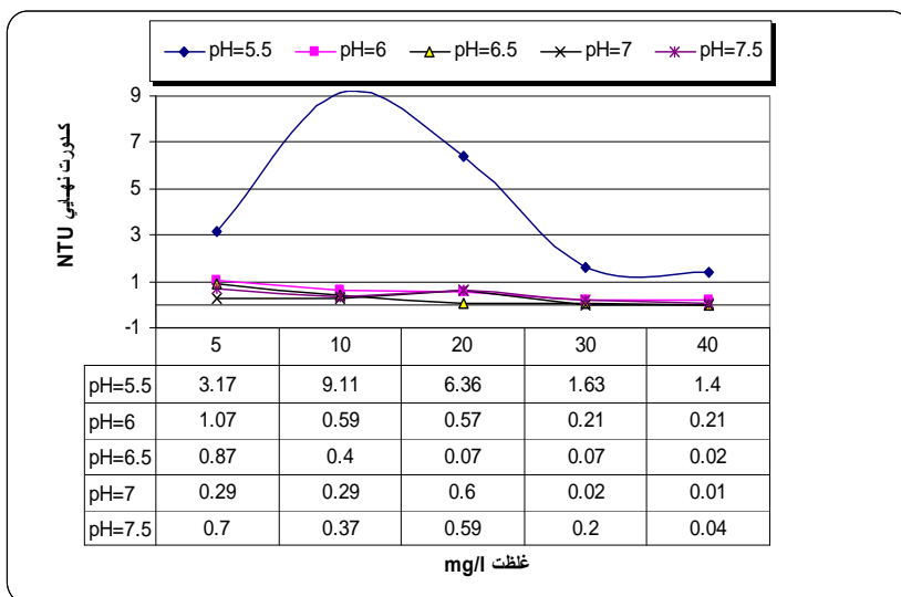
نمودار شماره ۴- کدورت نهایی در غلظت ها و pH های مختلف منعقد کننده کلراید فریک با کدورت اولیه ۸۰ NTU
